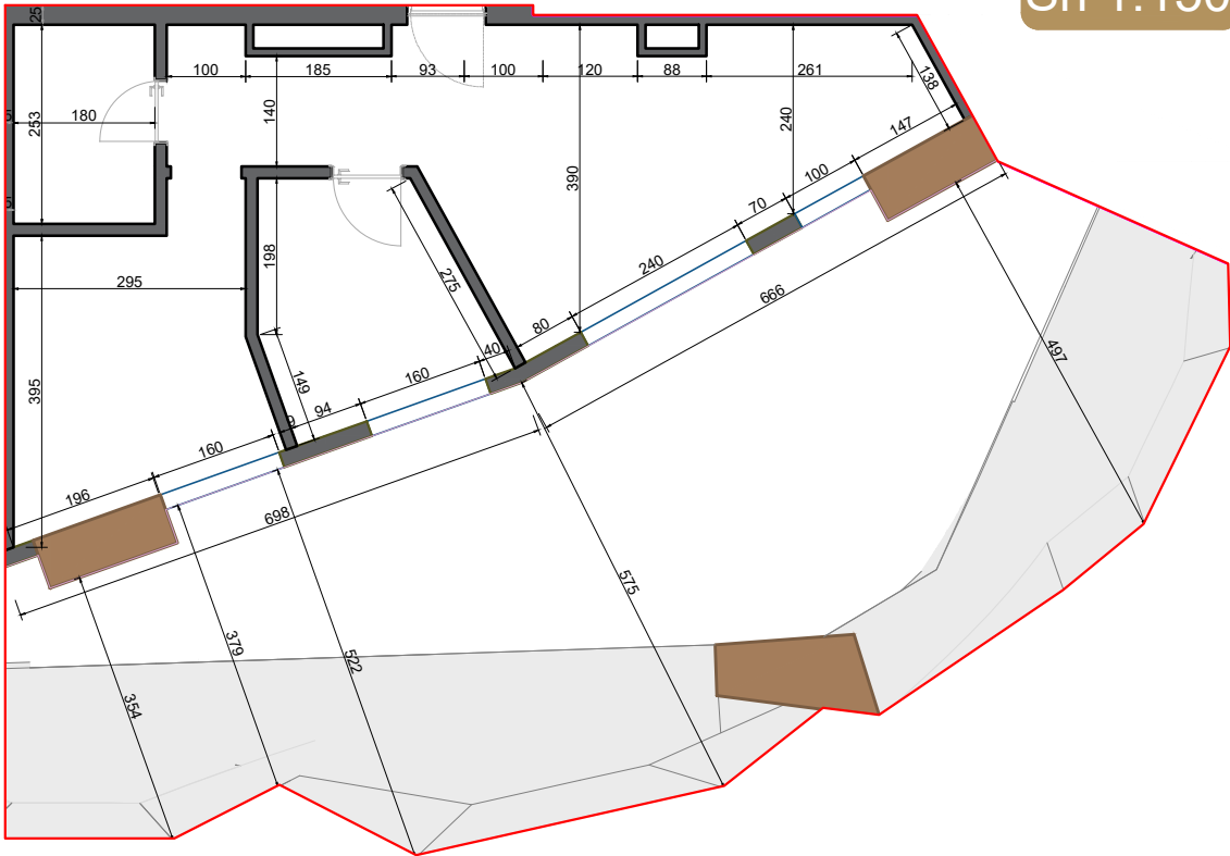
Plan dimensionimi
