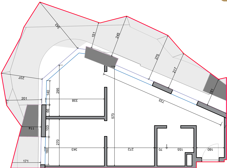
Plan dimensionimi
