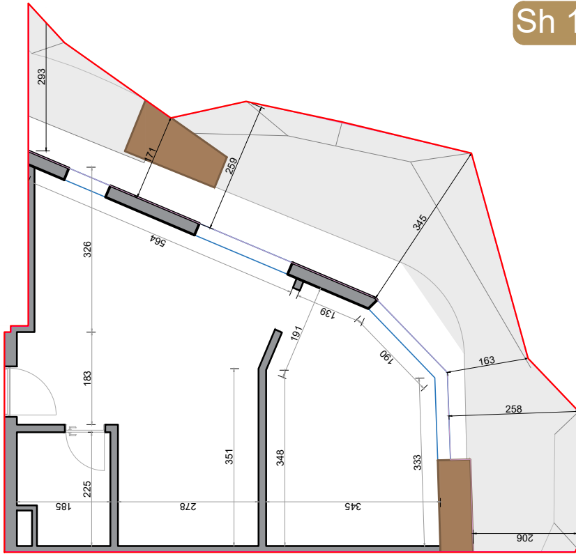
Plan dimensionimi
