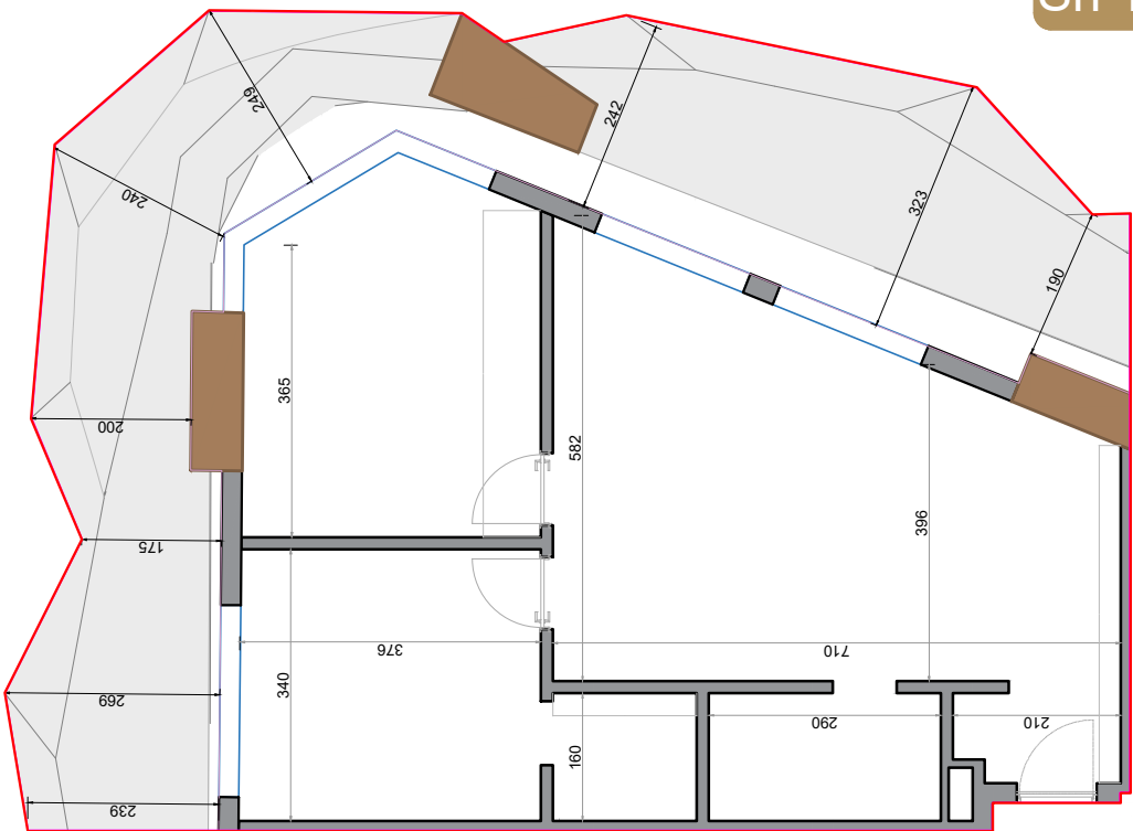
Plan dimensionimi
