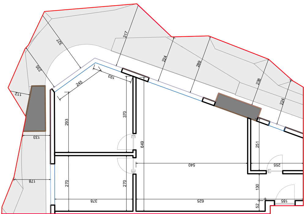
Plan dimensionimi
