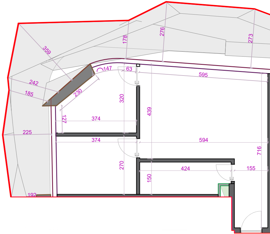
Plan dimensionimi
