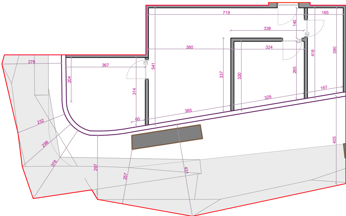
Plan dimensionimi
