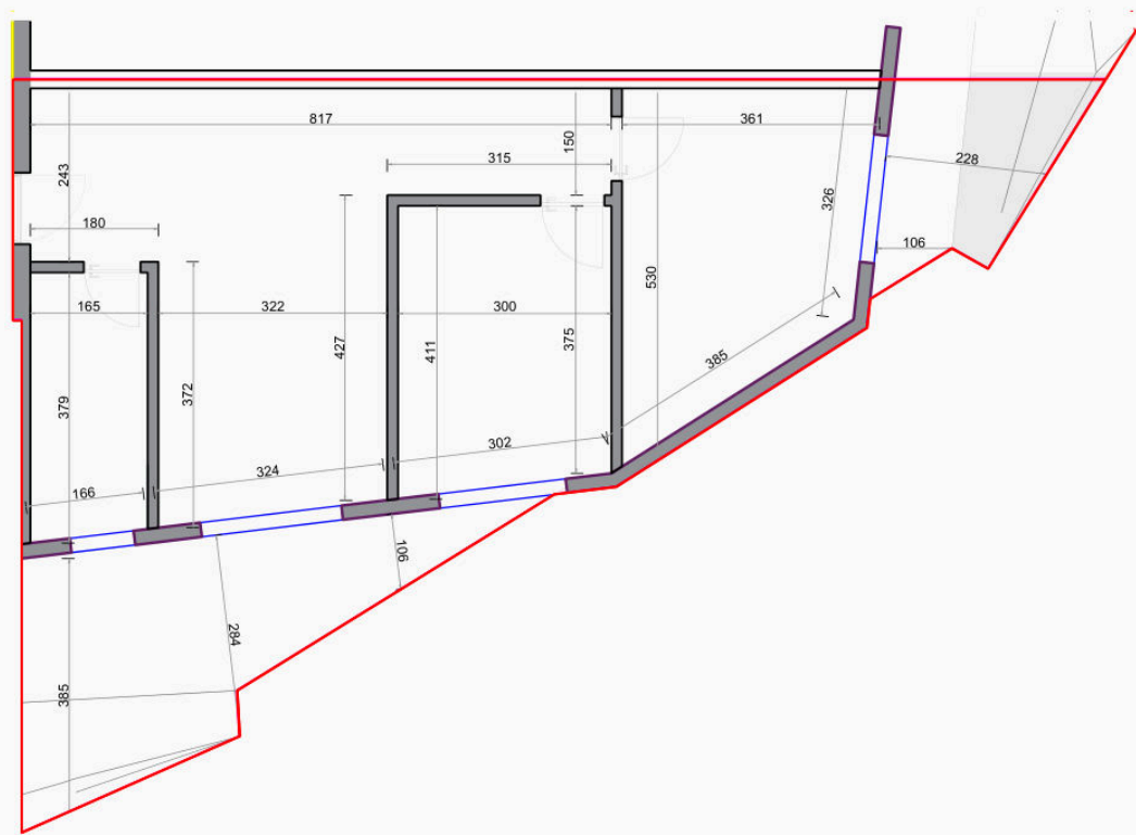
Plan Dimensionimi
