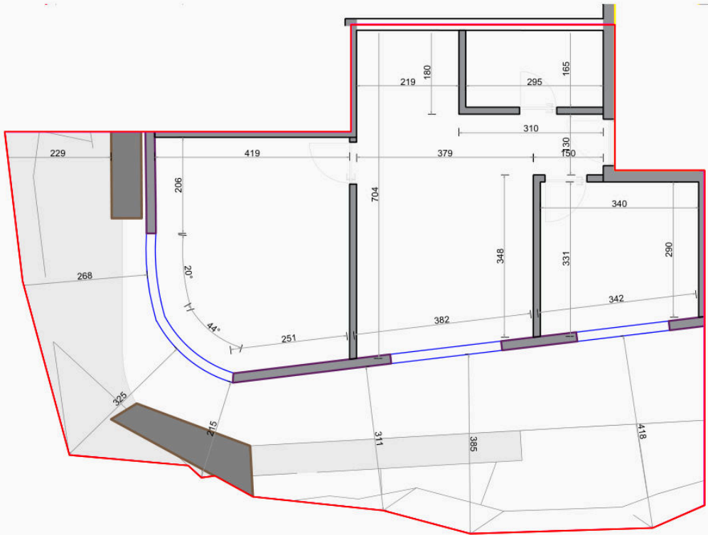
Plan Dimensionimi
