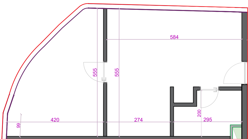
Plan dimensionimi
