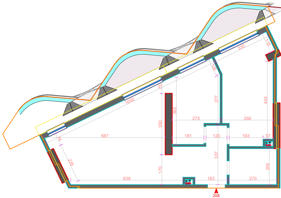
Plan Dimensionimi
