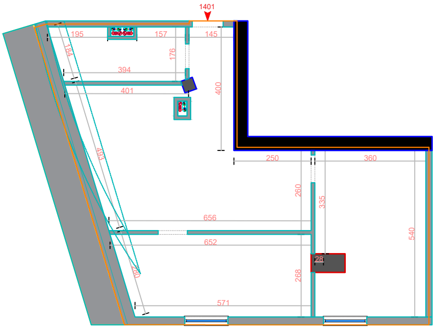
Plan Dimensionimi
