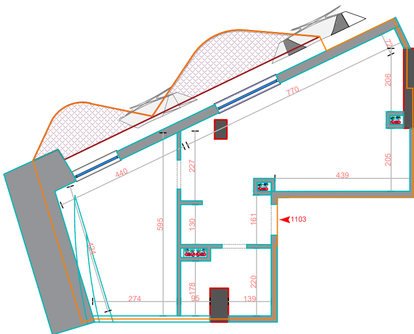
Plan Dimensionimi
