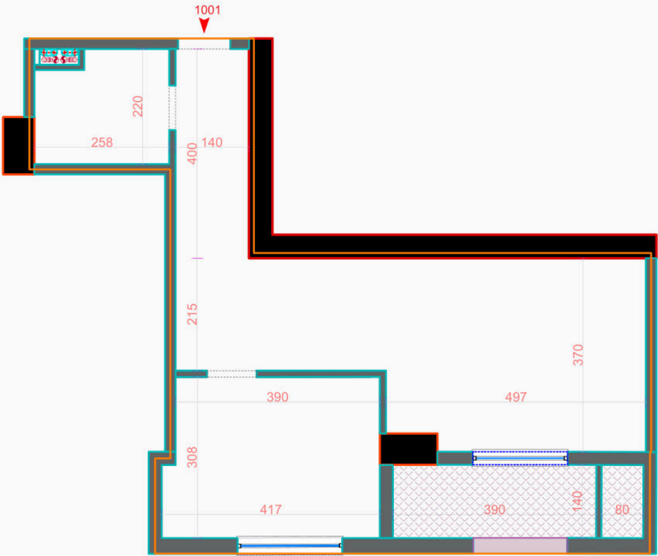
Plan Dimensionimi
