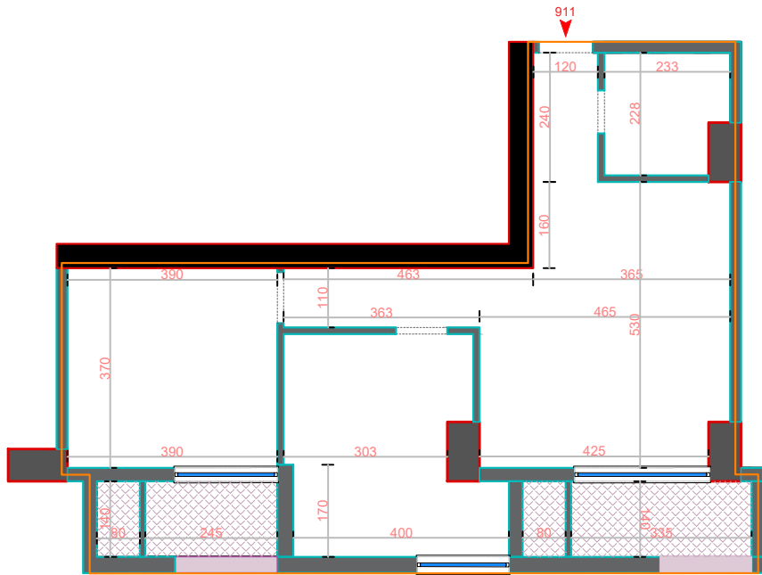
Plan Dimensionimi
