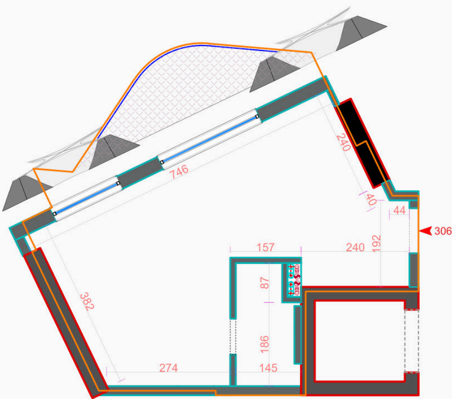
Plan Dimensionimi
