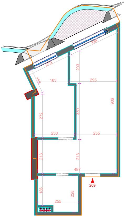
Plan Dimensionimi
