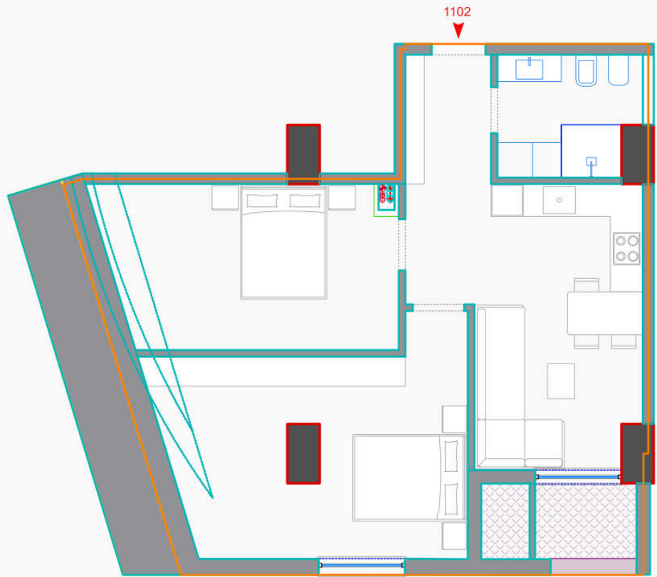
POZICIONIMI I APARTAMENTIT NË PLAN
