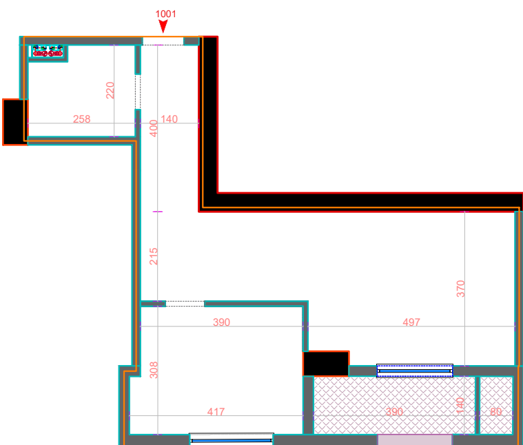
Plan Dimensionimi
